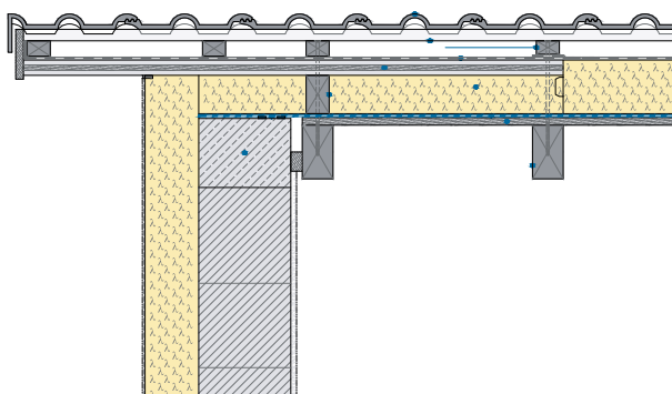
Obr. 30: Zakončení střechy na obvodové stěny
