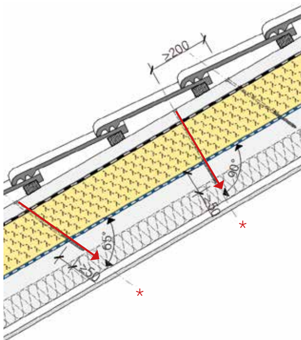
Obr. 33: Hloubka kotvení ≥ 50 - 75 mm (*)
