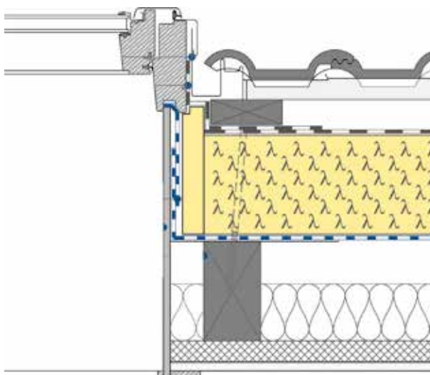
Obr. 36: Izolační rám (varianta 1)
