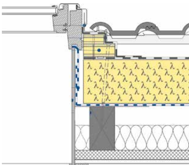
Obr. 37: Izolační rám PDZ (varianta 2)
