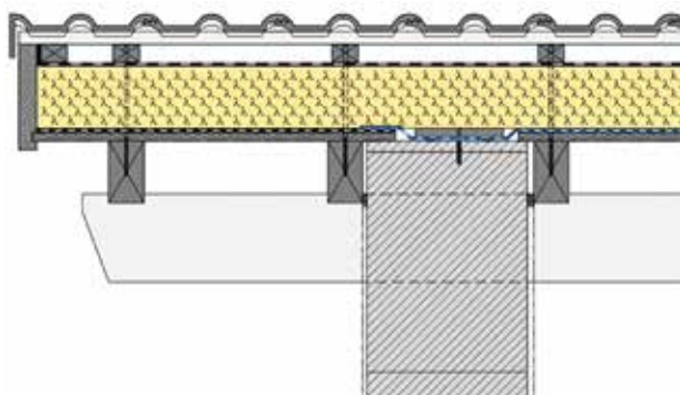
Obr. 29: Přesah střechy přes obvodovou stěnu
