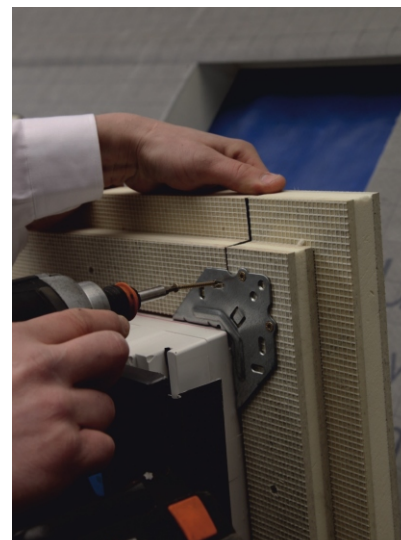
puren Dämmzarge PDZ - der optimale Eindeckrahmen für Dachflächenfenster. Winddicht, regensicher, biologisch und bauökologisch unbedenklich, unverrottbar, recycelbar, schimmel- und fäulnisfest. Lieferbar passend für die meisten handelsüblichen Dachfensterformate.
