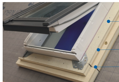
Ober- und Unterseite purenit - veredelttes Upcyclingprodukt auf PUR/PIR-Hartschaumbasis Kern aus Hochleistungsdämmstoff PUR/PIR-Hartschaum WLS 030 werkseitig ausgerüstet mit Kompriband für sichere Anschlüsse
